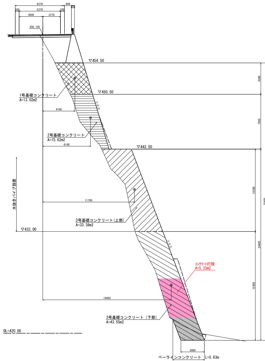
NO. 2+6.5 (起点) (ペーロケ断面)
